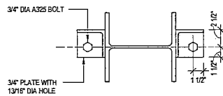
D1 DETAIL
